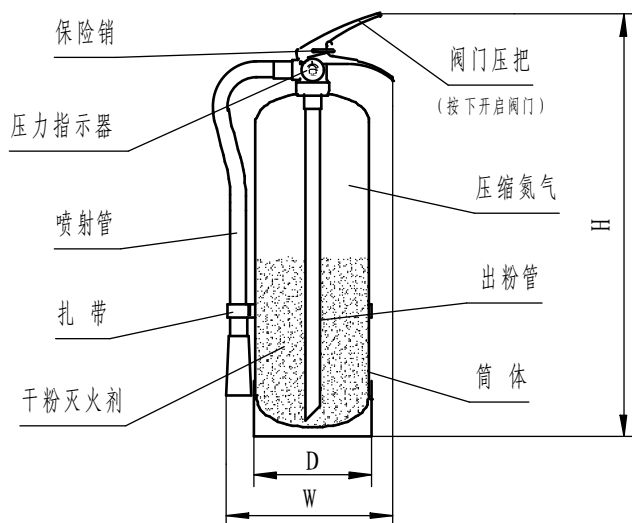
手提式干粉灭火器结构简图（1kg、2kg、3kg 无喷射管）
